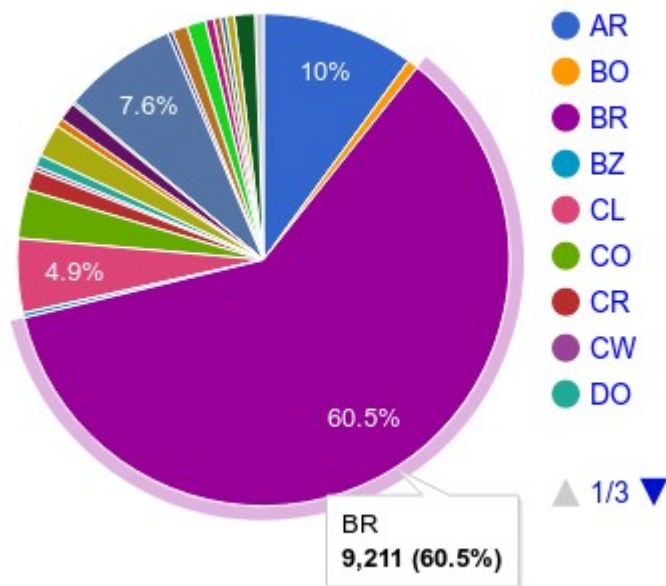
Distribuição de blocos IPv4 por país
